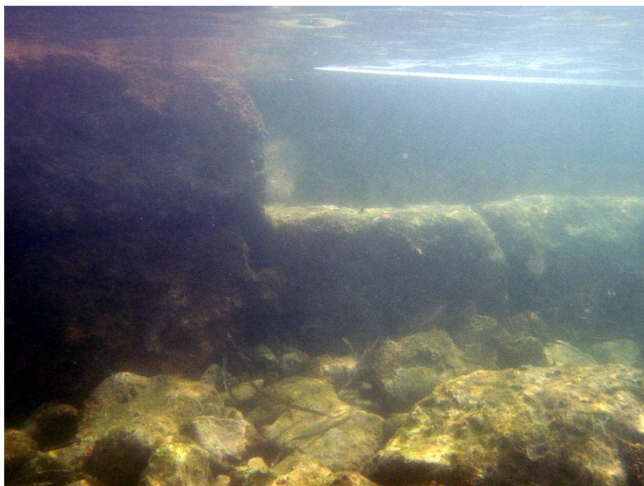
Εικόνα 3: Υποβρύχια λήψη από την πρόσοψη του κρηπιδώματος στην κορυφή του προσήνεμου ανατολικού λιμενοβραχίονα
