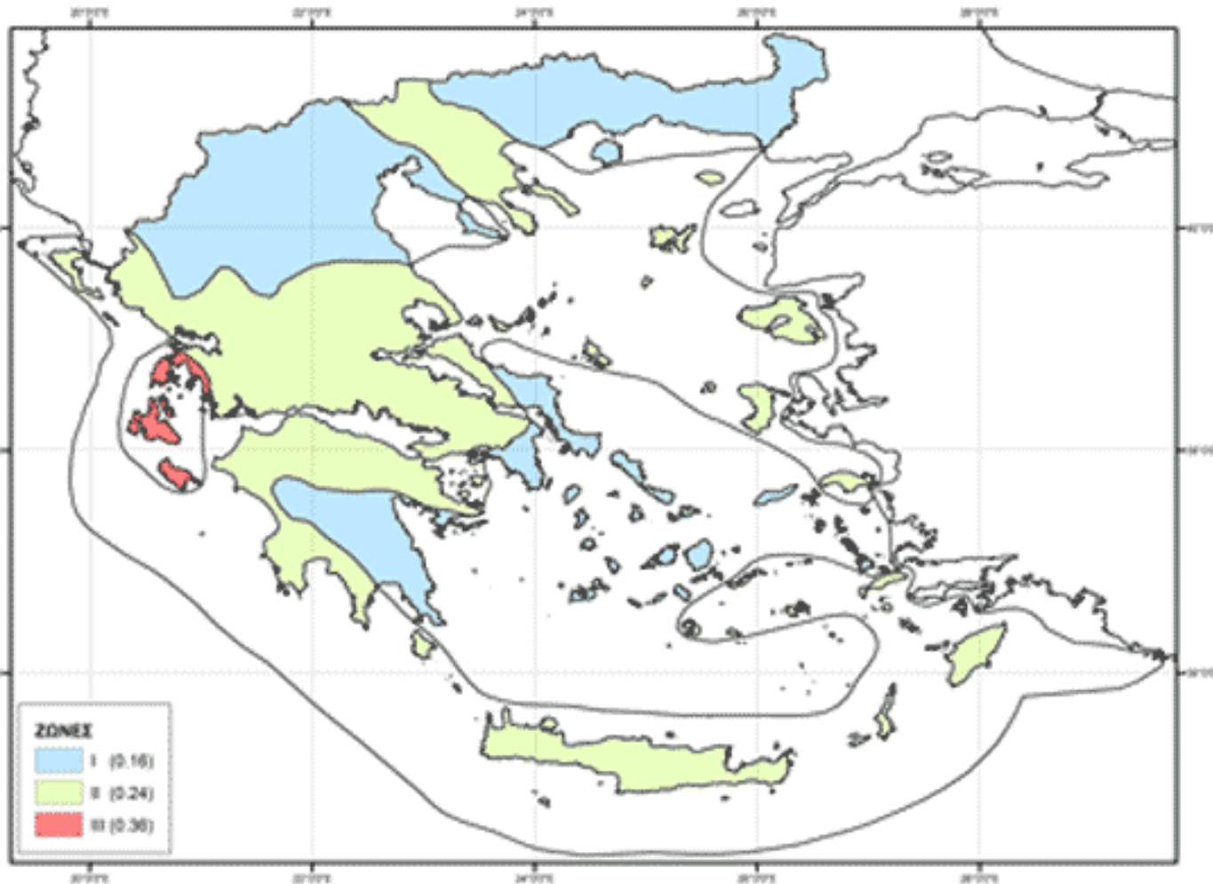
ΝΕΟΣ ΧΑΡΤΗΣ ΣΕΙΣΜΙΚΗΣ ΕΠΙΚΙΝΔΥΝΟΤΗΤΑΣ
